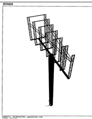
Imagen No. 5 – Estructura modelada, diseñada y calculada en los estudios técnicos y planos presentados. Tomada del radicado 2011ER122055 del 28/09/2011.
