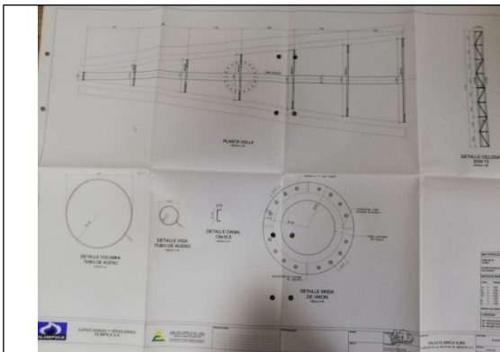
Imagen No. 1 – Foto tomada de los planos de la valla en planta adjuntos a la solicitud de registro nuevo, donde se muestran las cerchas, tubo horizontal y dos tableros publicitarios separados tipo en “V”
