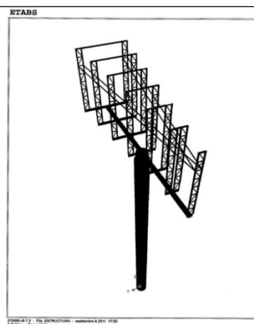
Imagen No. 4 – vista en 3D de la estructura de la valla diseñada. Tomada del radicado 2011ER122055 del 28/09/2011
