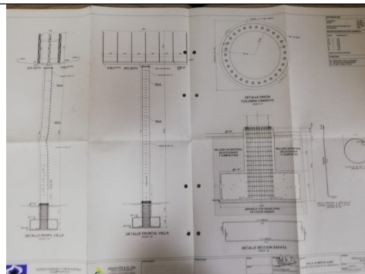
Imagen No. 2 – Planos en alzado de la valla donde se evidencia un tipo de estructura de mástil centrado.
