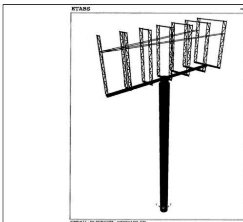
Imagen No. 3 – Modelo matemático generado para las memorias de cálculo estructural y análisis de estabilidad. Tomada del radicado 2011ER122055 del 28/09/2011
